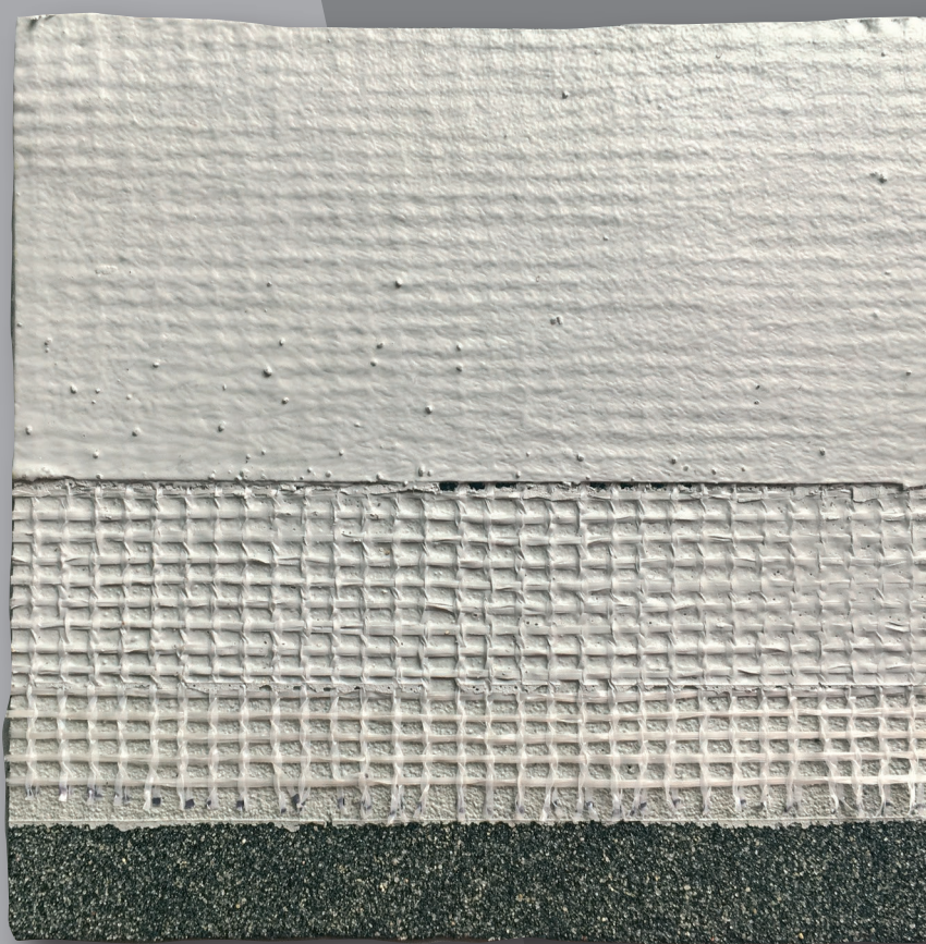
hydroizolační systém s výztužnou tkaninou
